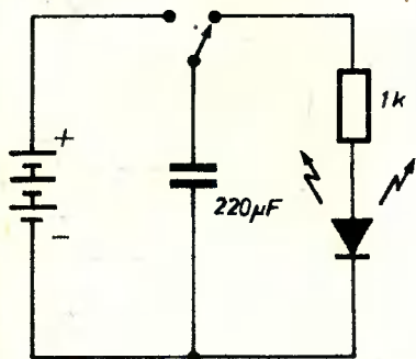
Рис. 3. Исследование емкости конденсатора в схеме со светящимся диодом: а — схема, б — внешний вид системы.
